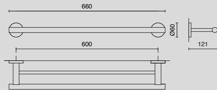
Doppel-Handtuchstange / double towel rail, Nr. 40 059
