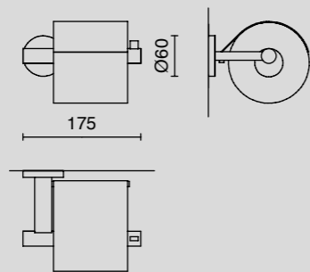
Toilettenpapierhalter / toilet roll holder Nr. 40 051
