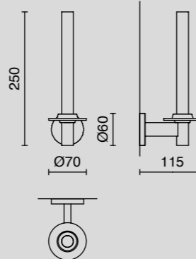
Ersatz-Toilettenpapierhalter / spare toilet roll holder, Nr. 40 053
