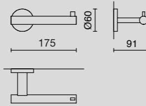
Toilettenpapierhalter / toilet roll holder Nr. 40 050
