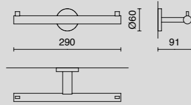
Doppel-Toilettenpapierhalter / double toilet roll holder, Nr. 40 052
