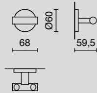
Doppel-Handtuchhaken / double towel hook, Nr. 40 063
