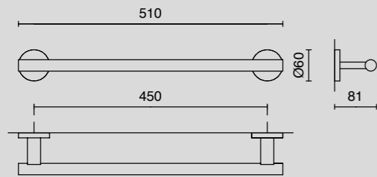
Handtuchstange / towel rail, Nr. 40 056 / Nr. 40 057 / Nr. 40 058
